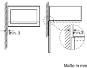
Mikrowelle Eckeinbau
