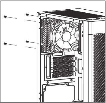
(6c) Install Rear Fan
