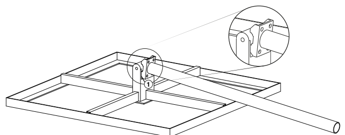
Abb. 2: Mast einsetzen
