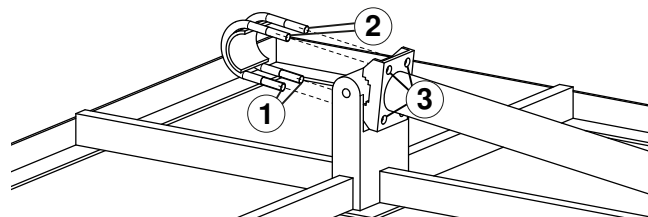
Abb. 3: Befestigungsbügel einsetzen
